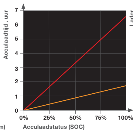
Acculaadtijd versus laadstatus (SOC)
