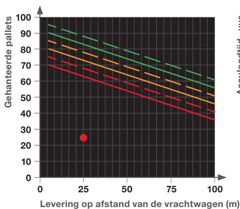
Accucapaciteit – gehanteerde pallets versus afstand
